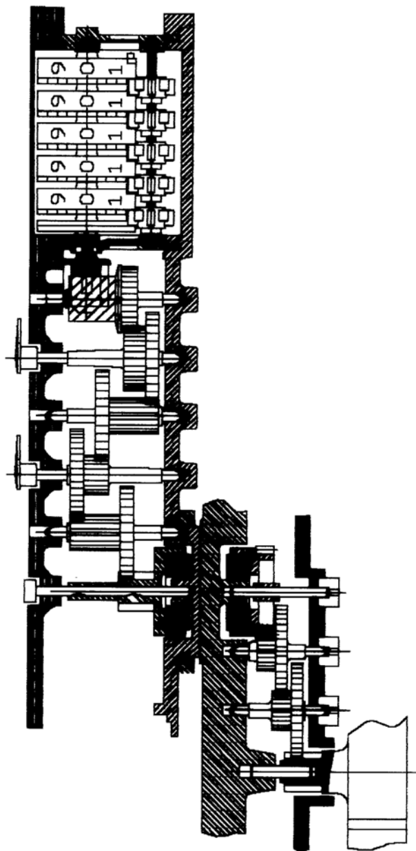
Detalhe Trem Redutor
