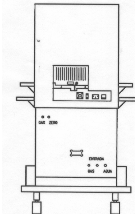
ANALISADOR DE GASES EC06010 - VISTA TRASEIRA.
