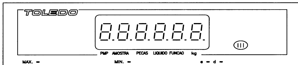
DISPOSITIVO INDICADOR DO OPERADOR, DISPLAY DUPLO E REMOTO
