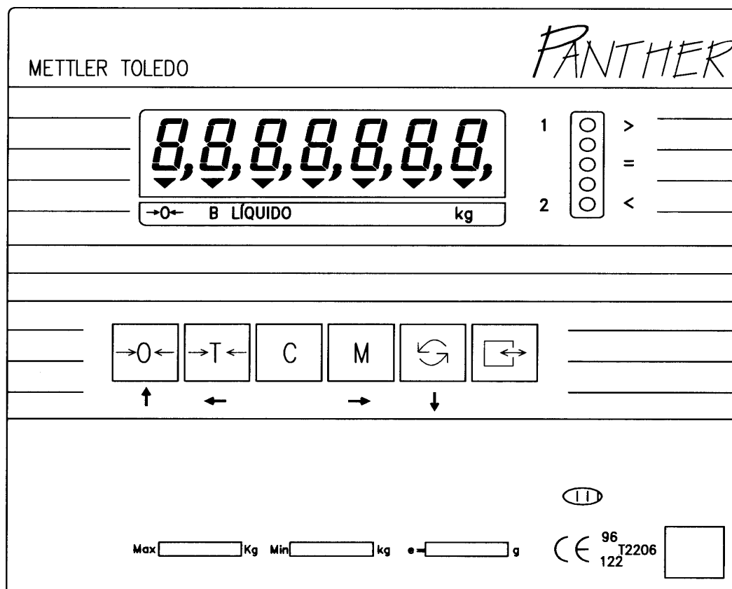
DISPOSITIVO INDICADOR E TECLADO
