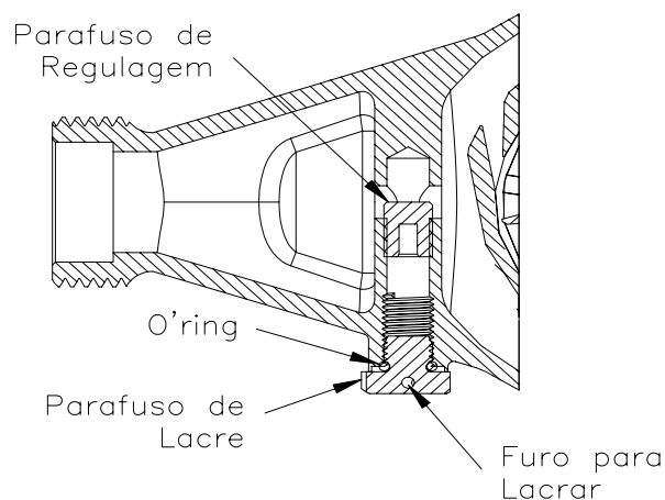
MECÂNISMO REGULADOR
