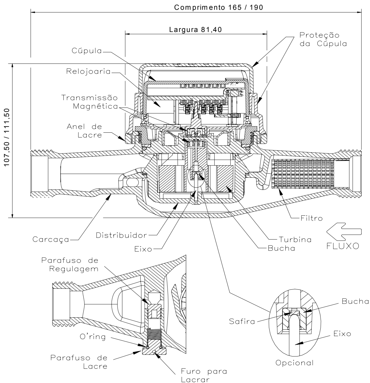
MECÂNISMO REGULADOR
