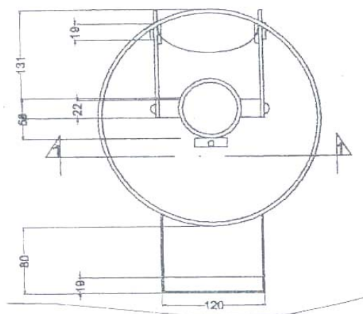
Vista Frontal Aferidor.
