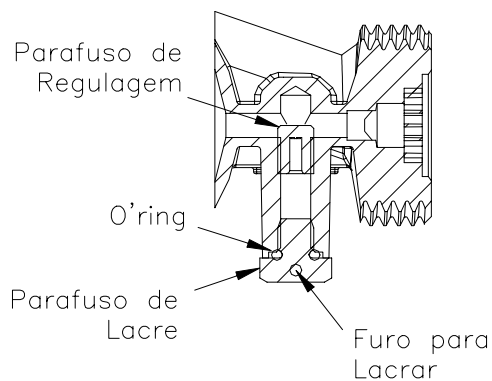
MECÂNISMO REGULADOR
