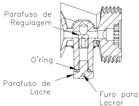
MECÂNISMO REGULADOR
