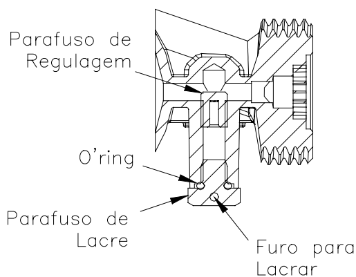
MECANISMO REGULADOR
