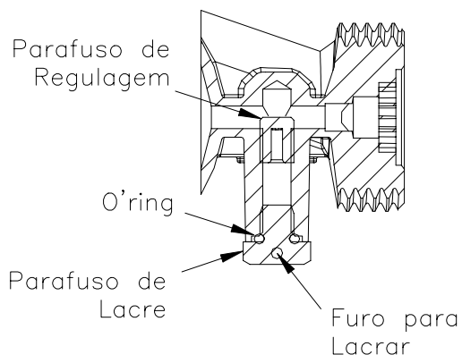
MECANISMO REGULADOR
