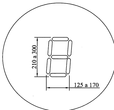
"DETALHE DO DÍGITO"
