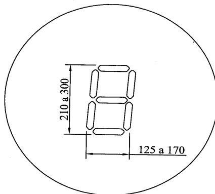
"DETALHE DO DÍGITO"
