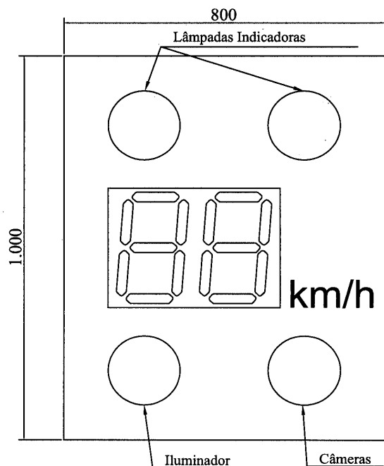
"Vista do Dispositivo Indicador 2 Dígitos"
