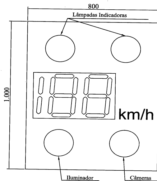
"Vista do Dispositivo Indicador 2 1/2 Dígitos"
