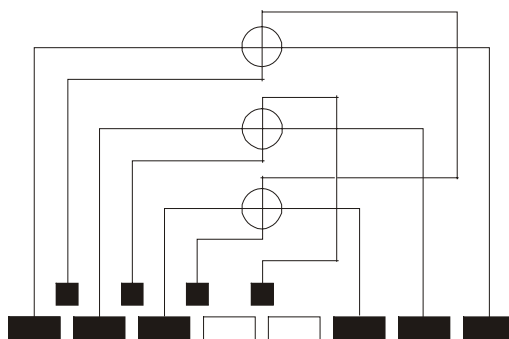
ESQUEMA DE LIGAÇÕES P/MEDIDOR 3 ELEMENTOS
