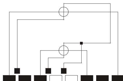
ESQUEMA DE LIGAÇÕES P/MEDIDOR 2 ELEMENTOS
