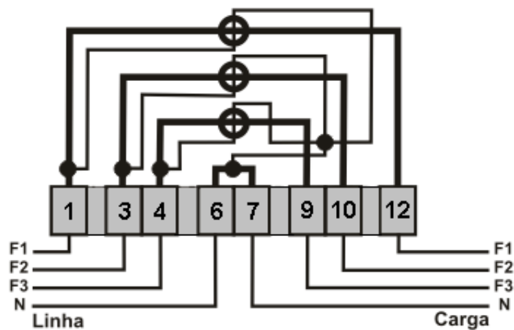
Ligação a 2 Elementos
