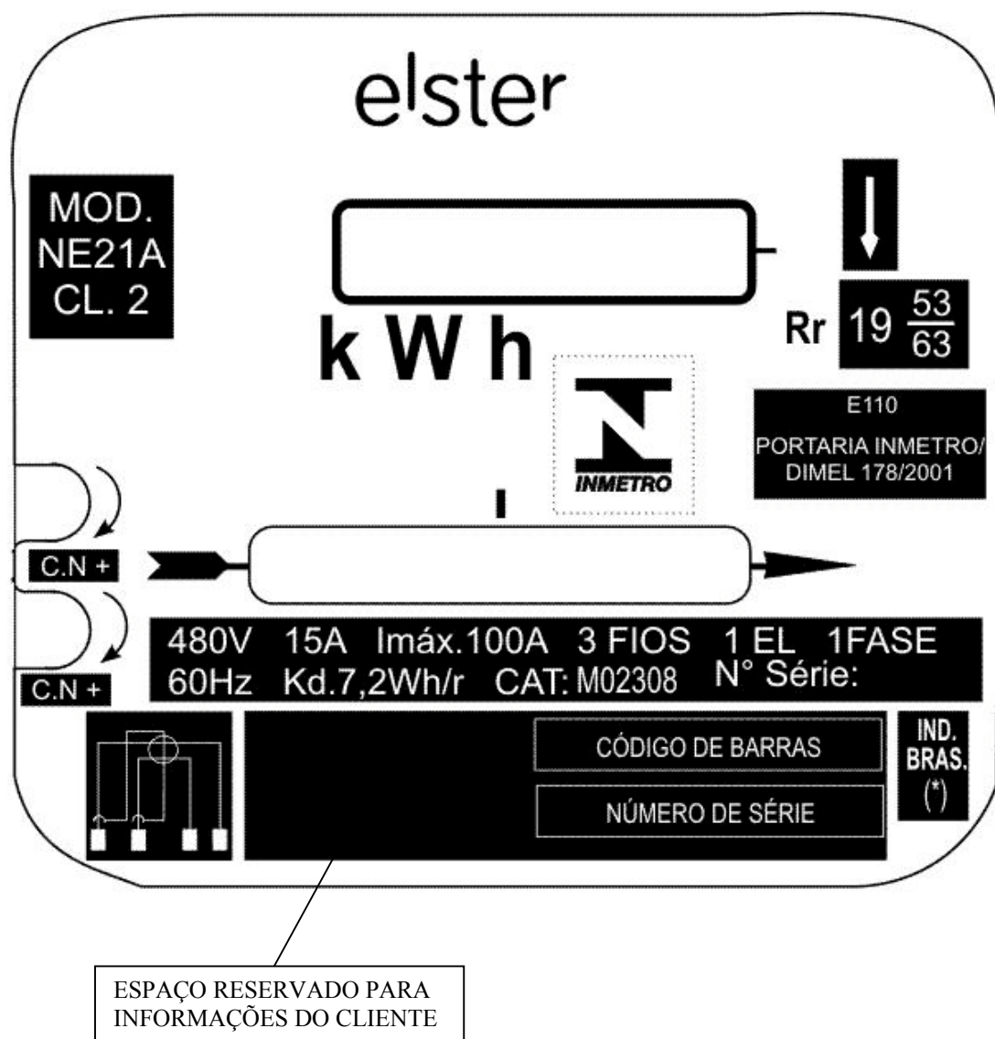
PLACA DE IDENTIFICAÇÃO EM 480 V
