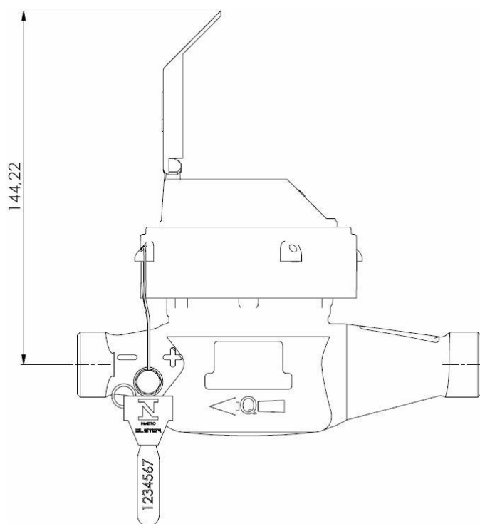
VISTA DE SELAGEM DO MEDIDOR MULTIJATO
