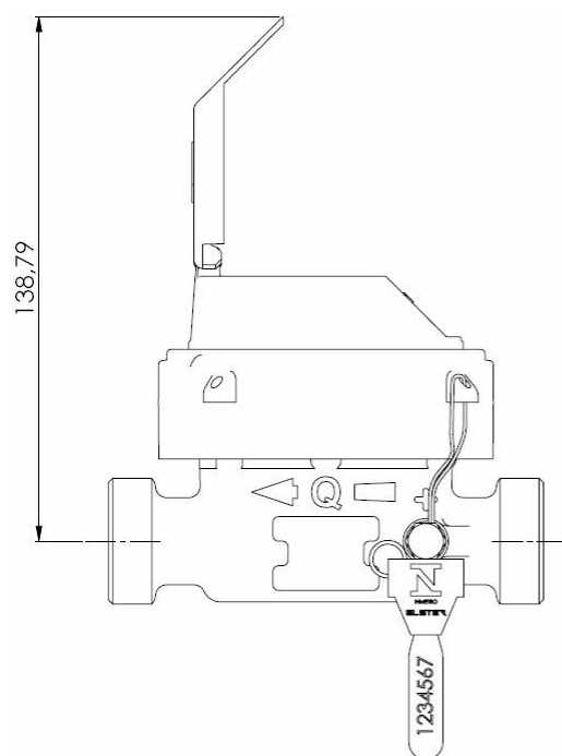
VISTA DE SELAGEM DO MEDIDOR UNIJATO
