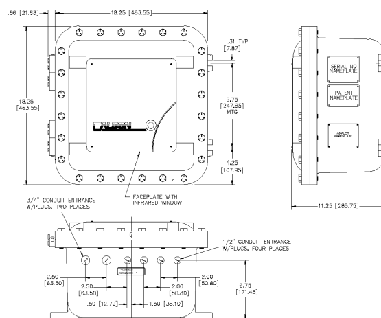
Transmissor Montado em Parede GP
