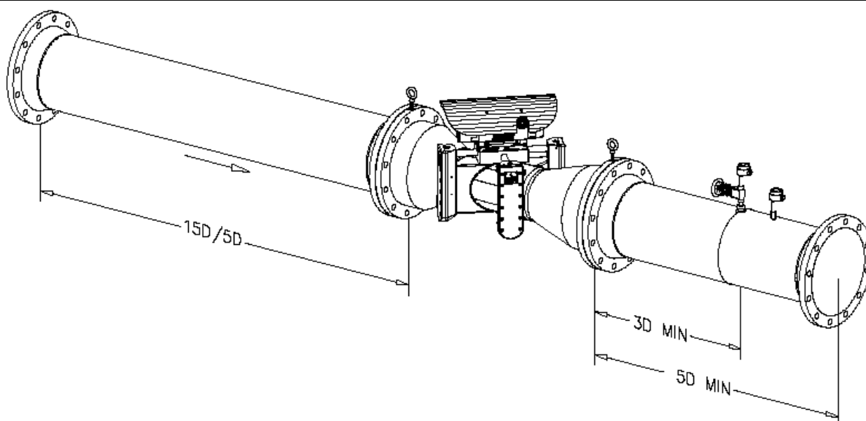
LEFM 280CiRN
