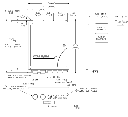
Transmissor Montado em Parede GP
