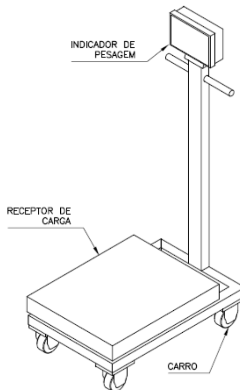
BALANÇA MODELO B COM CARRO
