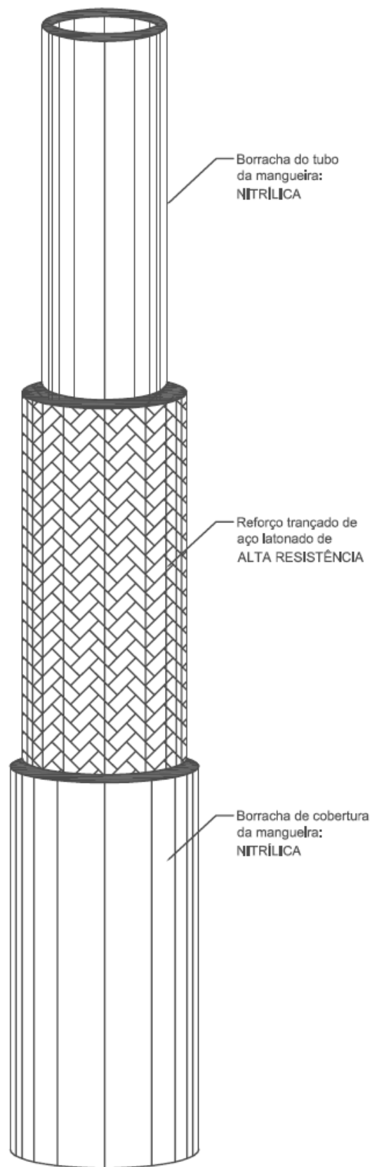
VISTA ESQUEMÁTICA
