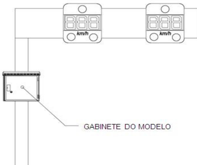
INSTALAÇÃO EM SEMIPIRTOCO OU ESTRUTURA EXISTENTE
